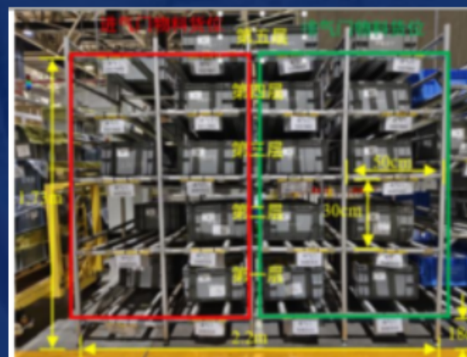
正视图尺寸
