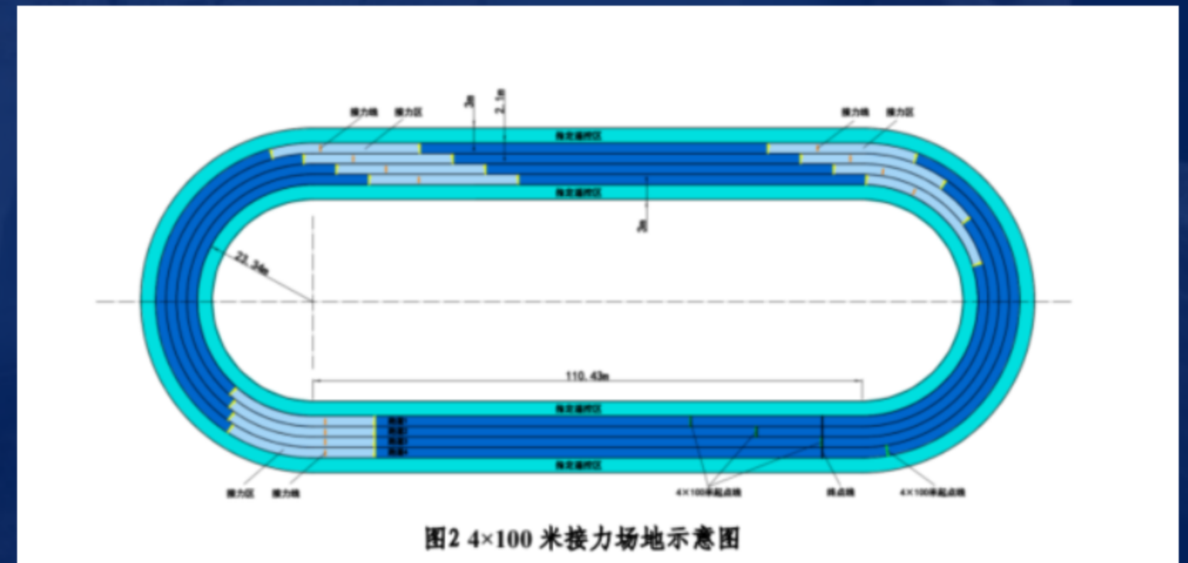
4 x 100m 계주 경기장
